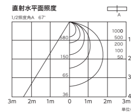
配光特性: MLSS-2-1000-N
