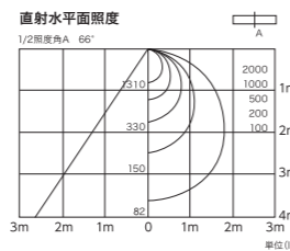
配光特性: MFSW-2-1000-N
